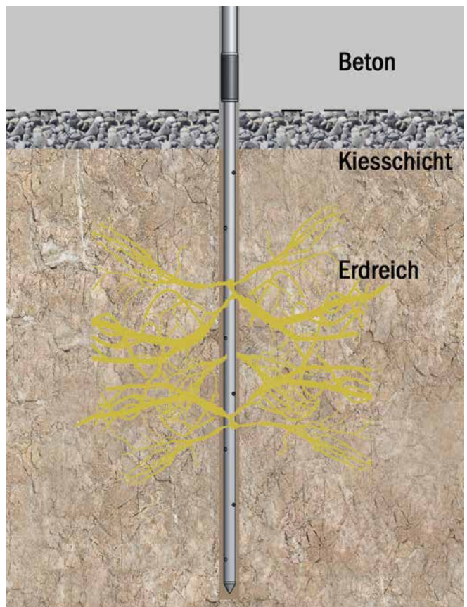
Anwendung von Rammverpresslanzen (Foto: Desoi)
