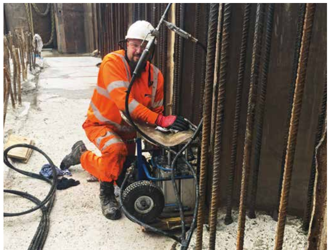
Abdichtungsinjektion mit RVL zwischen Bohrpfehl- und Spundwand
